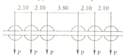
Схема нагрузки от электровоза ВЛ-22М
