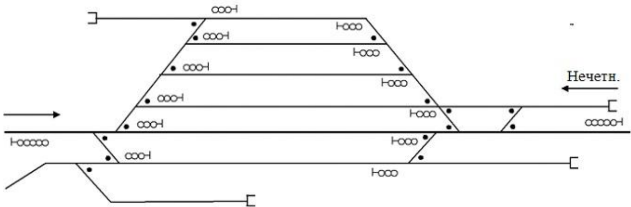
Рисунок 1 –Схема раздельного пункта для определения полной и полезной длины путей: I – главный (сквозной) путь, 2, 3, 4, 5, 6 – приемоотправочные пути, 7, 8, 9, 10 – тупиковые пути
